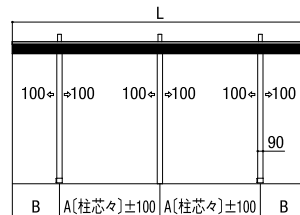
基本(W:33型) 側面図
