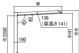
基本・縦2連棟 正面図
