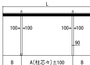
基本(W:24~30型) 側面図
