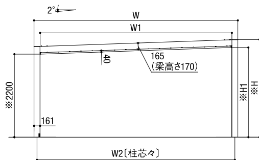
基本・縦2連棟 正面図
