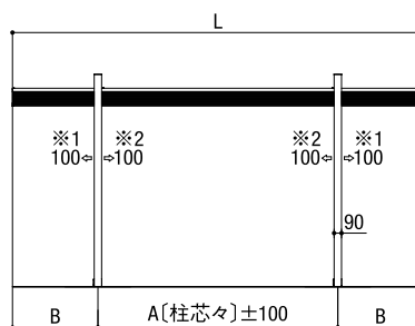
基本 (W:48~60型) 側面図
