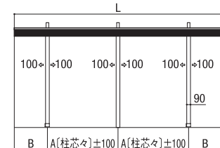
基本(W:33型) 側面図
