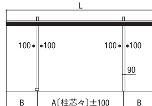
基本(W:24~30型) 側面図
